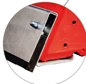
Sonderausrüstung "SOFT TOUCH" zusätzlich mit Klemmblech 4 mm und Gummi 2200 x 258 x 30 mm
